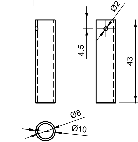
Cylindre laiton
