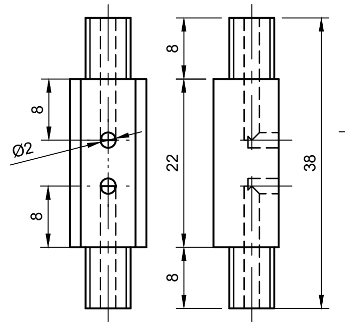
Cylindre laiton
