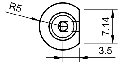
Alimentation vapeur - laiton Ech 2
