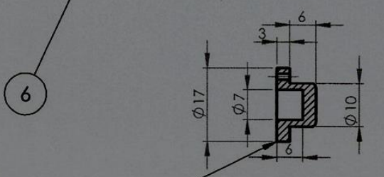
5 Doorsnede C-C achterwielkap
