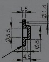
Doorsnede D-D voorwielkap
