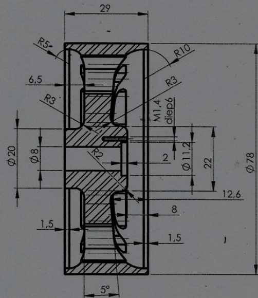
Doorsnede B-B
