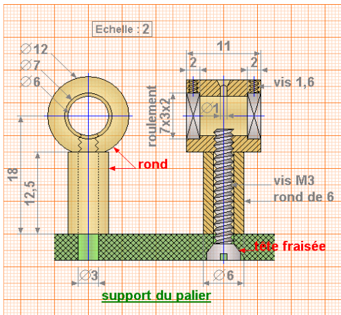
support de palier
