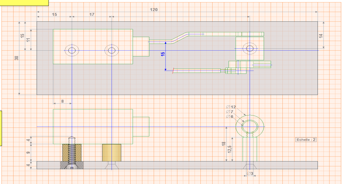
support de palier
