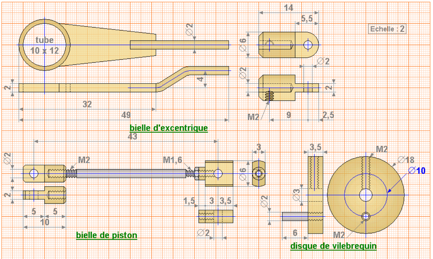
bielles, disque de vilebrequin
